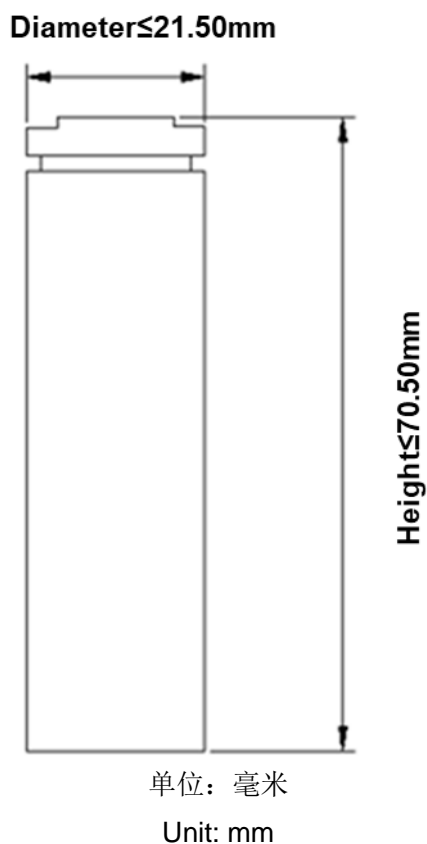
图 1:INR21700-40XG 电芯的外形尺寸
