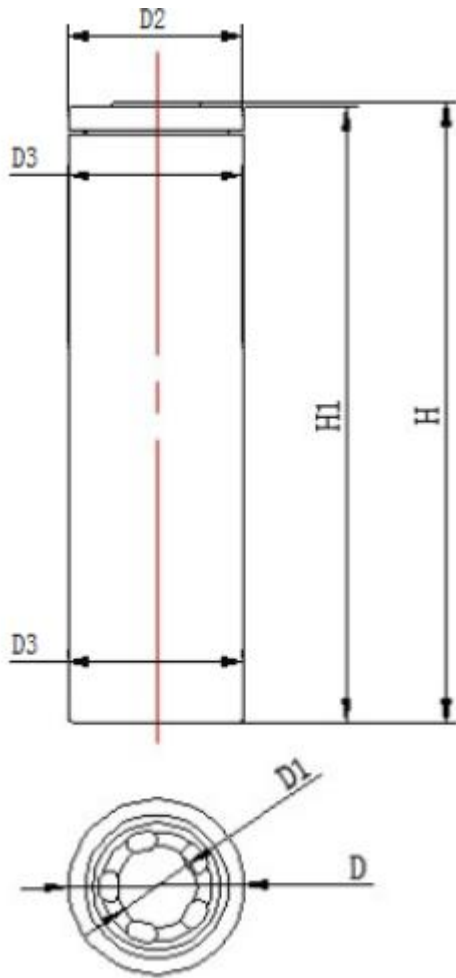
电芯外型尺寸图
