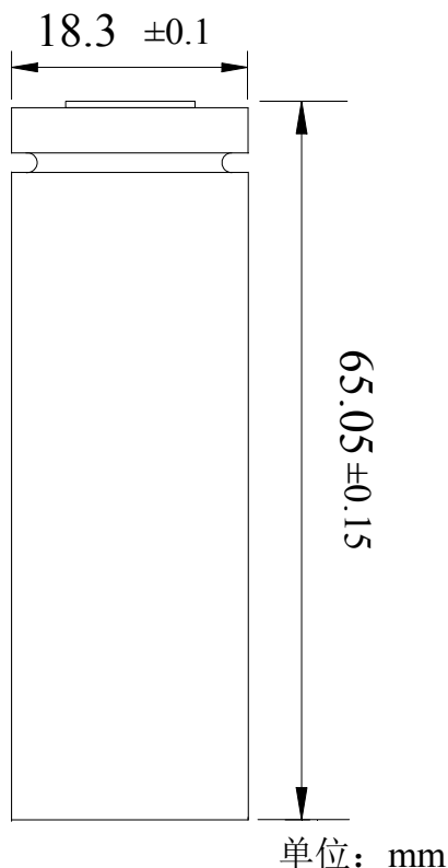
图 1 CMICR18650F5-2200mAh 电芯的尺寸示例图 (尺寸含套膜)
